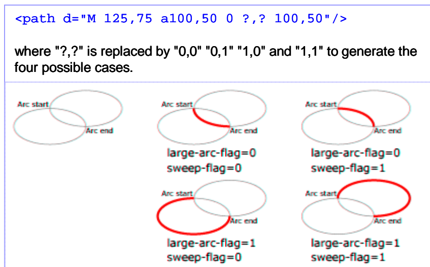
Abb. 6 Definition eines elliptischen Bogens in SVG
